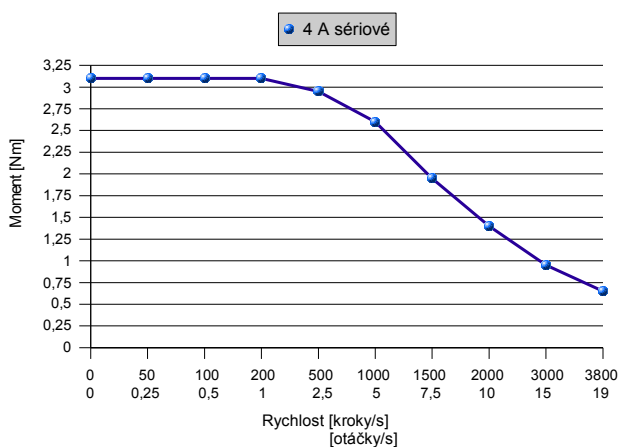
Momentová charakteristika motoru SX24-3341 s jednotkami CD40x, CD40M a napájecím napětím 48 VDC
