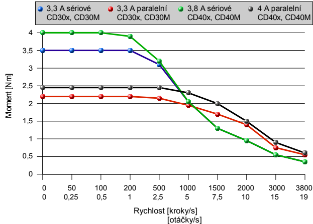
Momentová charakteristika motoru SX34-2740N s jednotkami CD30x, CD30M, CD40x, CD40M a napájecím napětím 48 VDC
